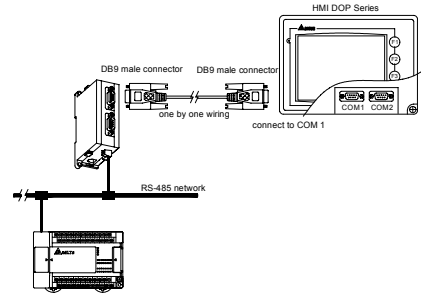
ADP485-01 ⇔ DOP (HMI)
