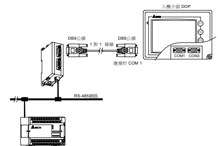
ADP485-01 ⇔ DOP 人機介面
